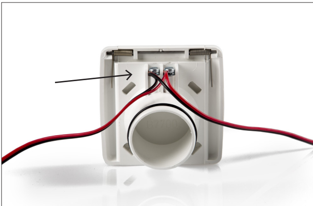
Achterkant van de vacuümaansluiting met 12V parallel connecties
