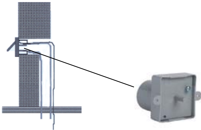
Gerader Millennium-Anschluß mit Putzschutz
